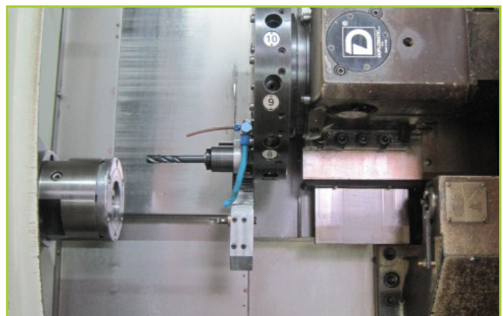
WEMAS ZPS 842 CNC/ 1999 CNC-DREHMASCHINE
