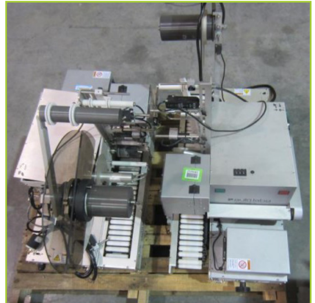
(3) AUTO-LABE 390 LABELER
